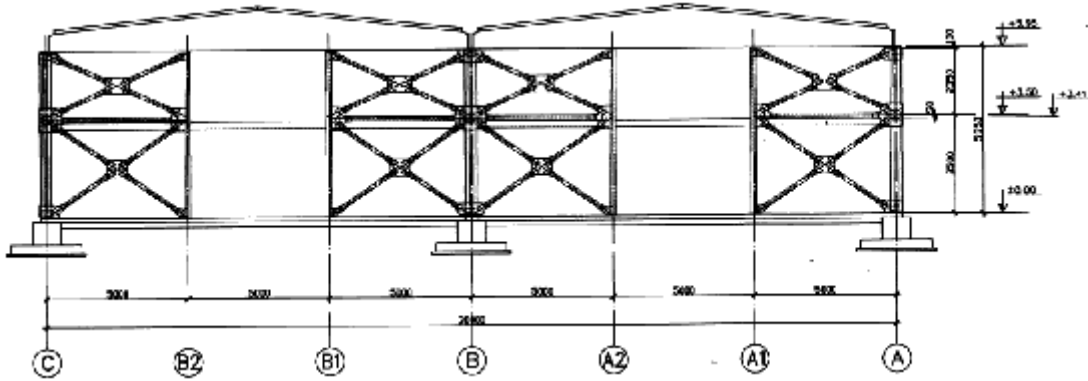
Resim 1. Çelik Çapraz Sistem İyileştirme Örneği
